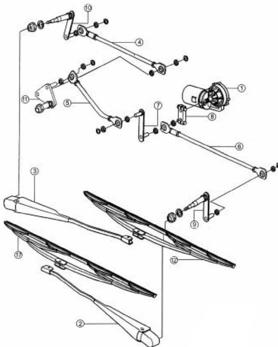
Torkarsystem B1 Bosch
