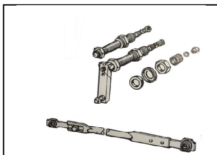
Torkarlager Vä 460310 Hjälplager Vä 460312 Länkstång 460318
